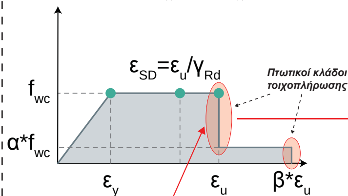
Σκελετικό διάγραμμα ενισχυμένης τοιχοπλήρωσης
