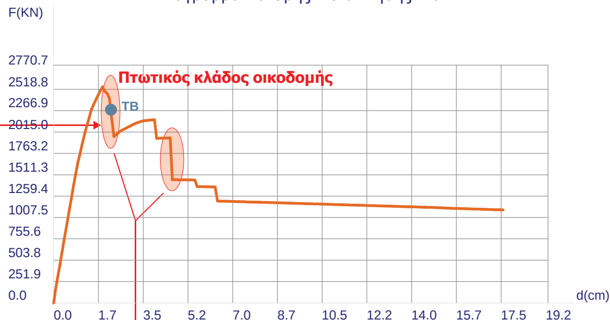
Διάγραμμα Δύναμης-Μετακίνησης F-d
