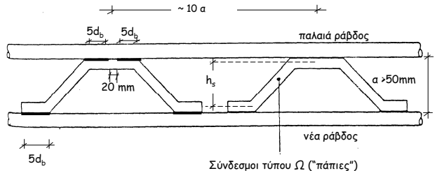
ΕΥΚΑΜΠΤΟΙ ΣΥΝΔΕΣΜΟΙ
