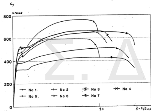
Διαγράμματα τάσεων παραμορφώσεων δοκιμασθέντων χαλύβων” 29 (Τζωρτζάκης κ.α., 1990)
