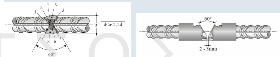
Διαδοχική εκτέλεση κορδονιών και πάσων Μετωπική σύνδεση με υποστήριγμα της ρίζας της συγκόλλησης
