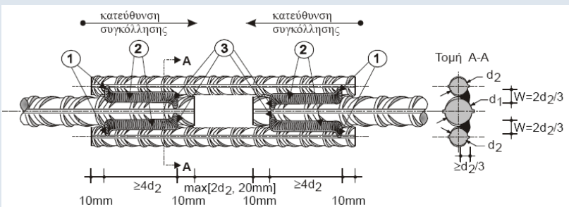
Σύνδεση με λωρίδες (Κ.Τ.Χ. 2007)
