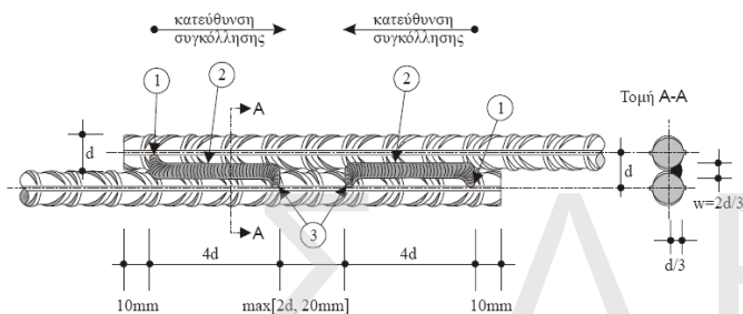
Σύνδεση κατά παράθεση με τεχνικές τόξου (Κ.Τ.Χ. 2007)
