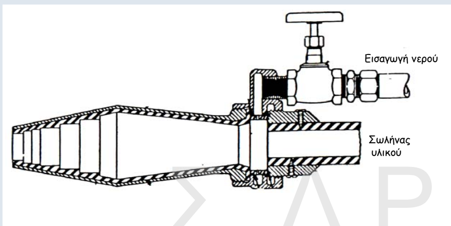
Τομή Ακροφυσίου
