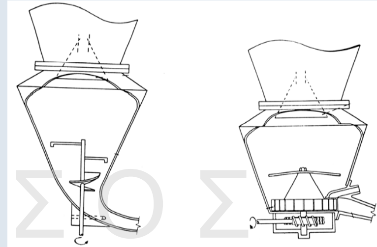
Σχηματικές Τομές Ενόσ Τύπου Μηχανής Προώθησης
