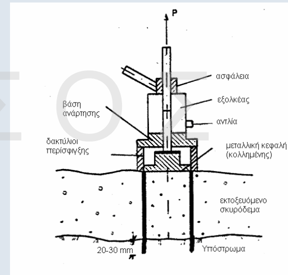
Εργαστηριακός Έλεγχος Συνάφειας επί τόπου του έργου με διαχωρισμό δείγματος
