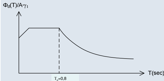
Σχήμα 1: Φάσμα σχεδιασμού
