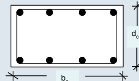
Σχήμα 2: Διαστάσεις διατομής
